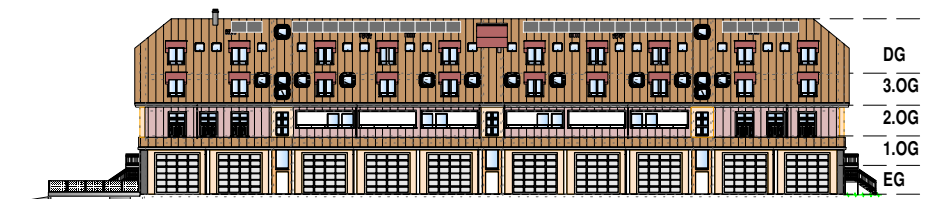
Ansicht Ost
