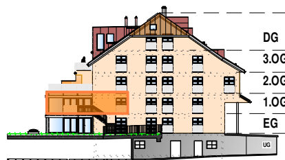
Ansicht Süd
