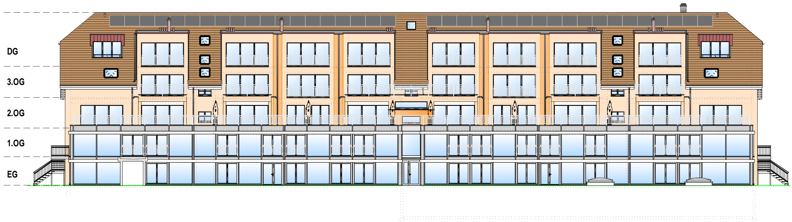
Ansicht West
